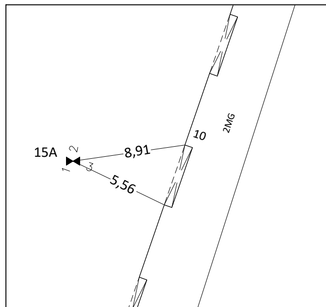
Prižišimo schema
