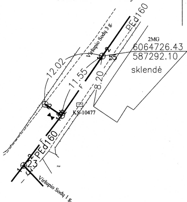
Pririšimo brėžinys
