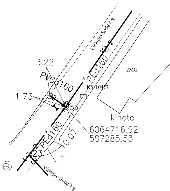
Pririšimo brėžinys
