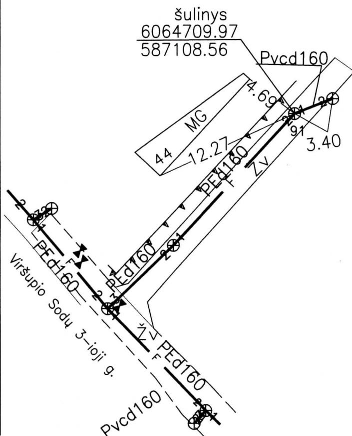
Pririšimo brėžinys
