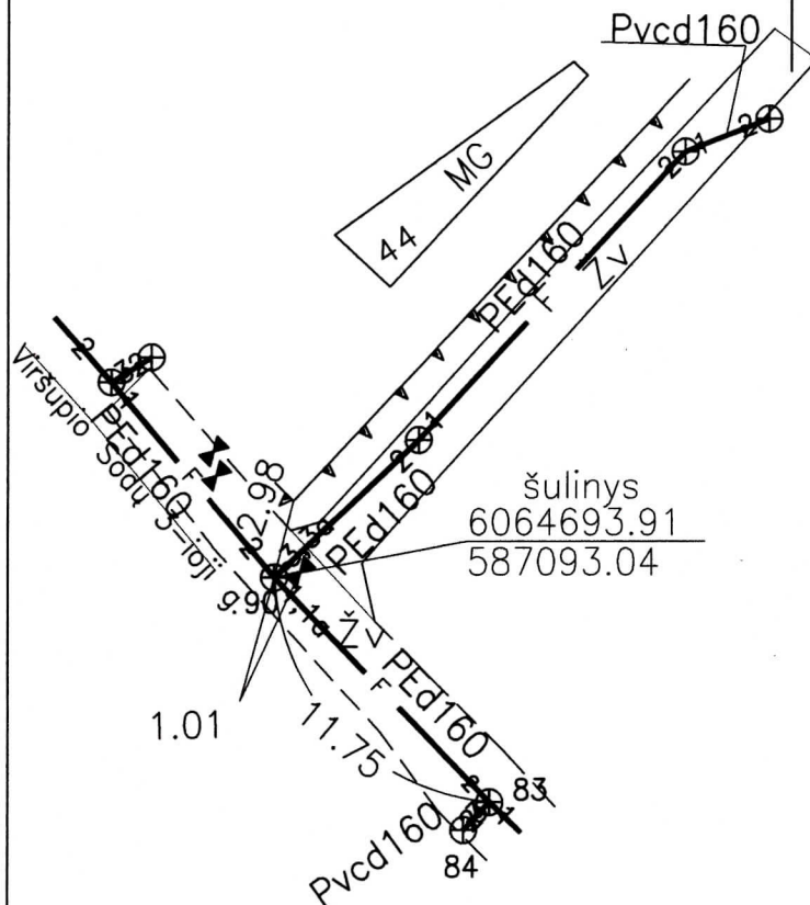
Pririšimo brėžinys
