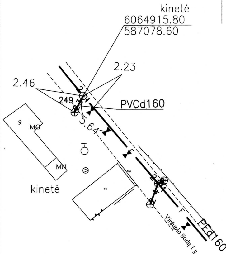
Pririšimo brėžinys
