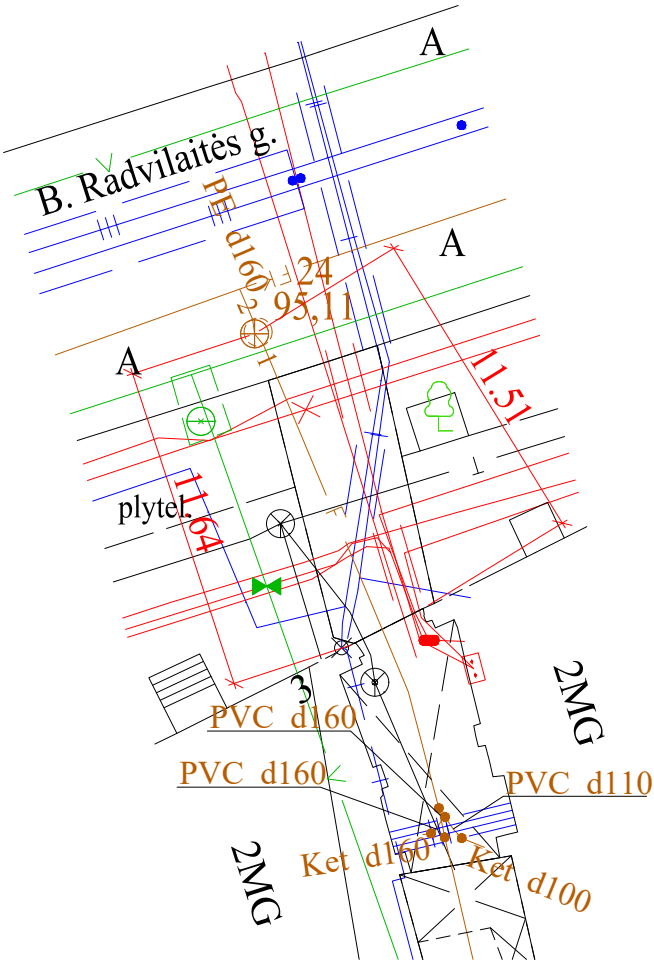
PRIRIŠIMO SCHEMA
