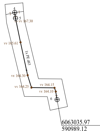
Priirišimo brėžinys :
