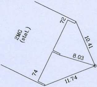
Pririšimo schema
