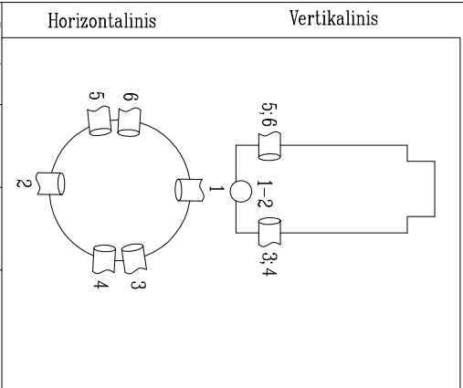
ŠULINIO PŪVIALAI (Matmenys duoti m)
