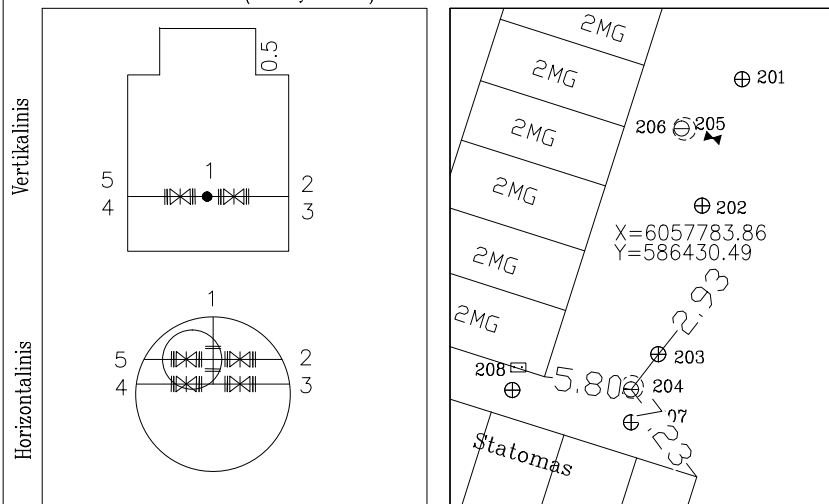
PRIRIŠIMO BRĖŽINYS
