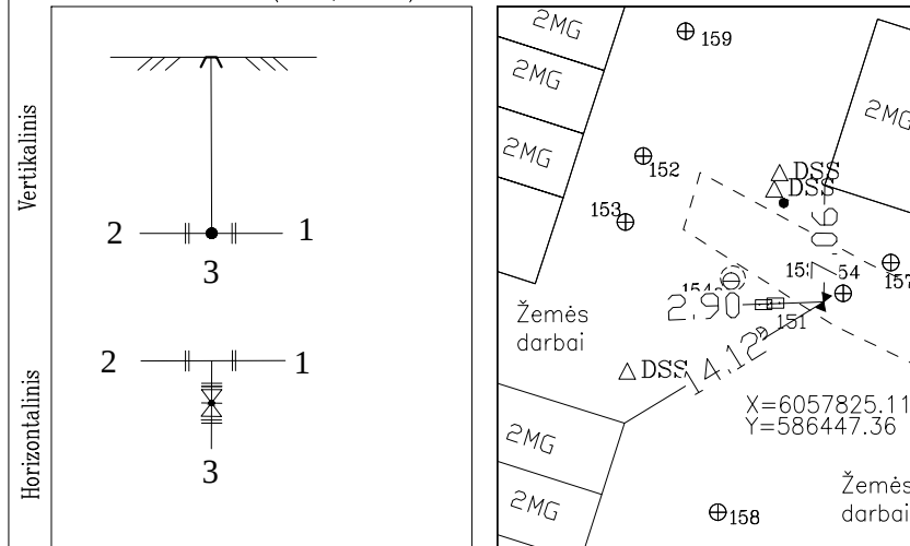
PRIRIŠIMO BRĖŽINYS
