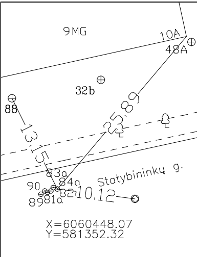
PRIRĖSIMO BRĖŽINYS
