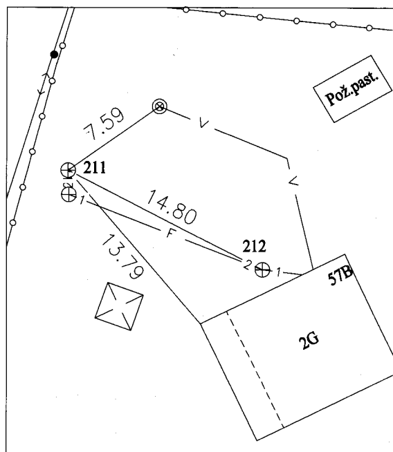
Pririšimo schema
