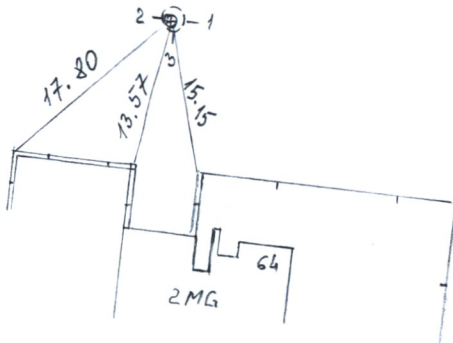
PRIRIŠIMO SCHEMA
