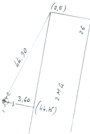
PRIRIŠIMO SCHEMA
