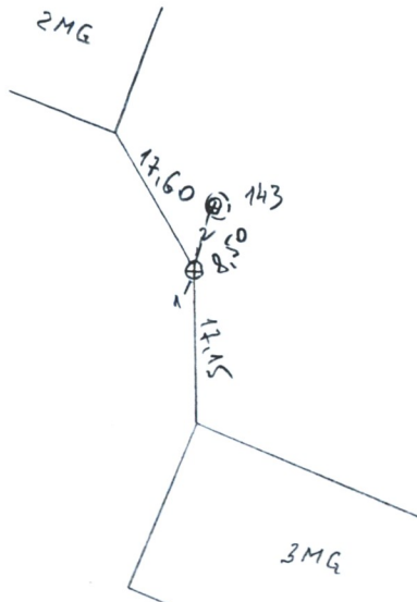
PRIRIŠIMO SCHEMA
