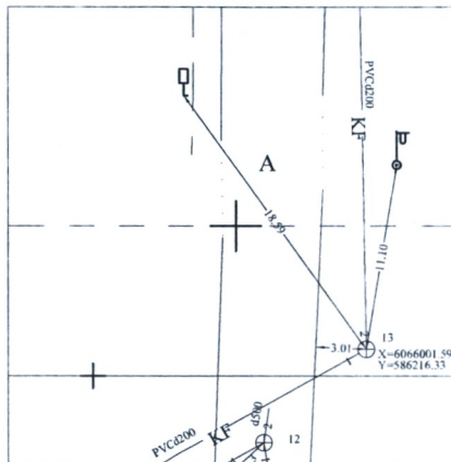
Sąsajos brėžinys
