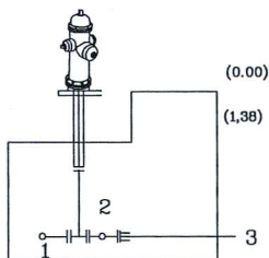
Šulinio pjūviai
