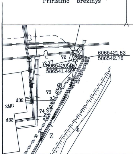
Pririšimo brėžinys
