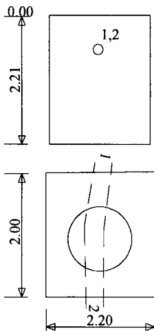
Šulinio pjūviai
