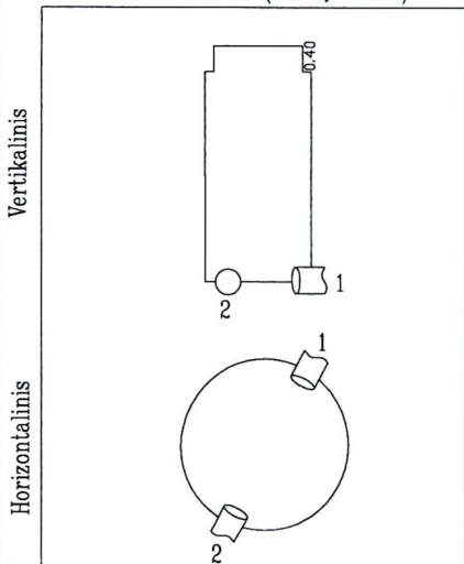
ŠULINIO PĖJŪVAI (Matmenys duoti m)
