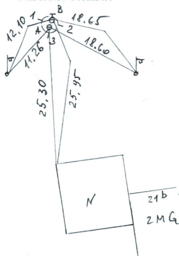
PRIRIŠIMO SCHEMA
