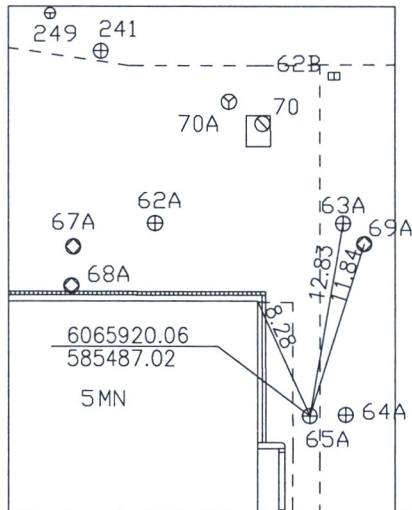
PRIRIŠIMO BRĖŽINYS
