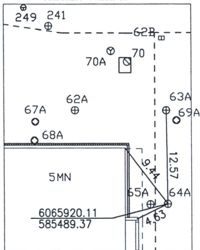
PRIRIŠIMO BRĖŽINYS
