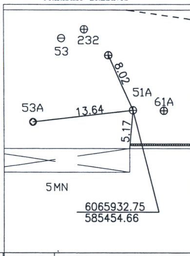
PRIRIŠIMO BRĖŽINYS
