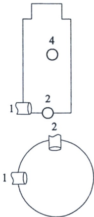
ŠULINIO PJŪVIAI (Matmenys duoti m)
