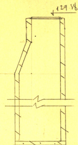
Чертеж колодца М 1:50
