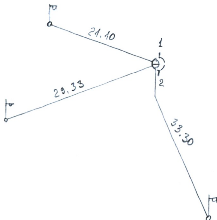
PRIRIŠIMO SCHEMA
