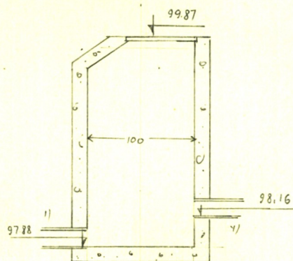
Чертеж колодца М 1:50
