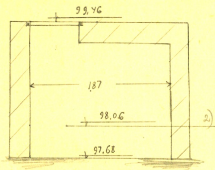
Чертеж колодца М. 1:50
