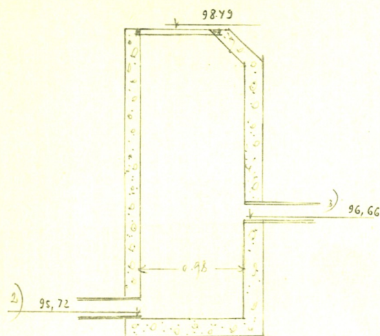
Чертеж колодца М 1:50
