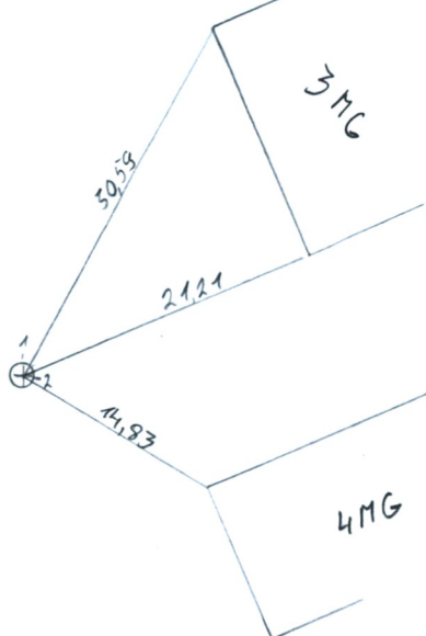
Pririšimo brėžinys
