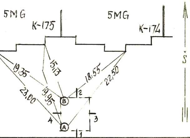
PRIRIŠIMO BRĖŽINYS:
