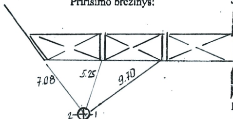
Pririšimo brėžinys:
