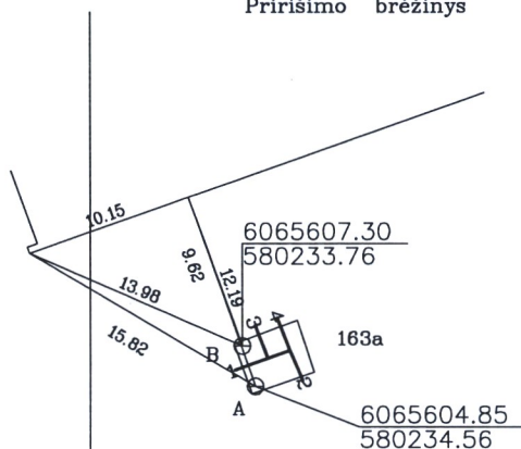
Pririšimo brėžinys
