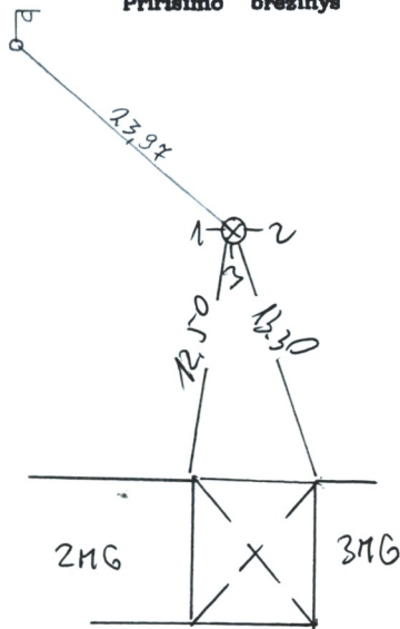
Pririšimo brėžinys
