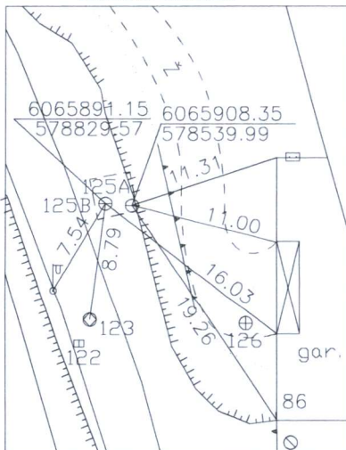
PRIRIŠIMO BRĖŽINYS
