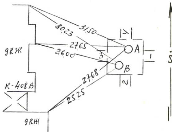
PRIRIŠIMO BRĖŽINYS:
