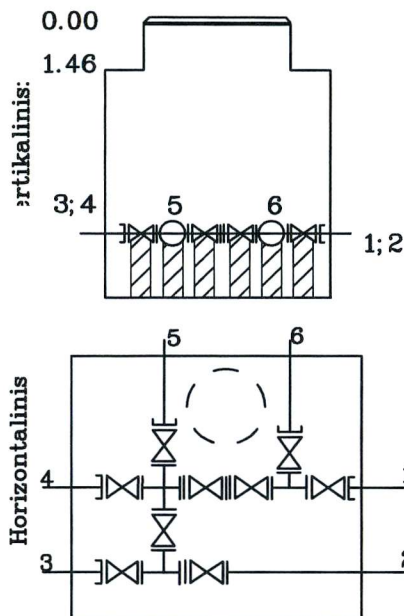
Šulinio pjūviai:
