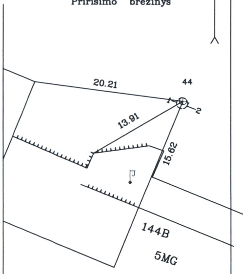
Pririšimo brėžinys
