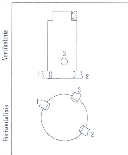
SULINIO PJŪVIAI (Matmenys duoti m)
