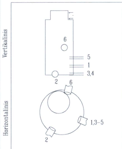
ŠULINIO PĖJŲVAI (Matmenys duoti m)
