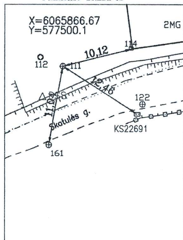
PRIRIŠIMO BRĖŽINYS
