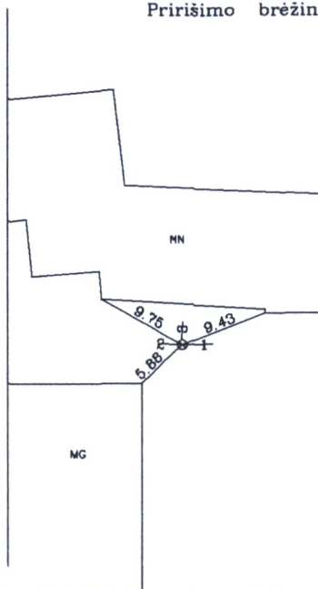
Pririšimo brėžinys
