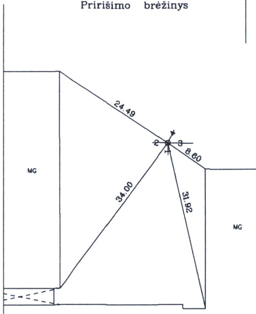
Pririšimo brėžinys
