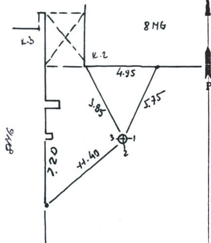
Pririšimo brėžinys:
