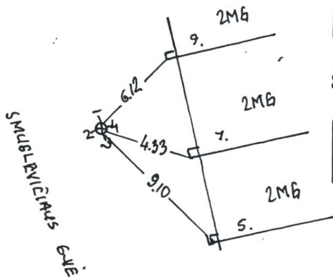
PRIRIŠIMO SCHEMA
