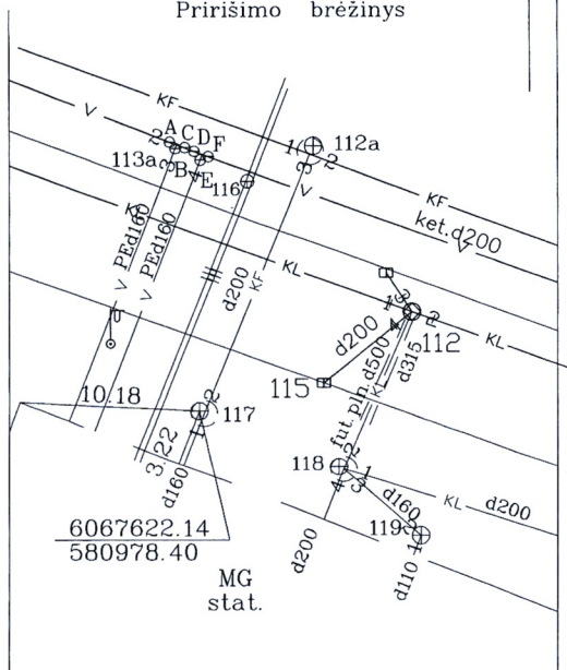
Pririšimo brėžinys
