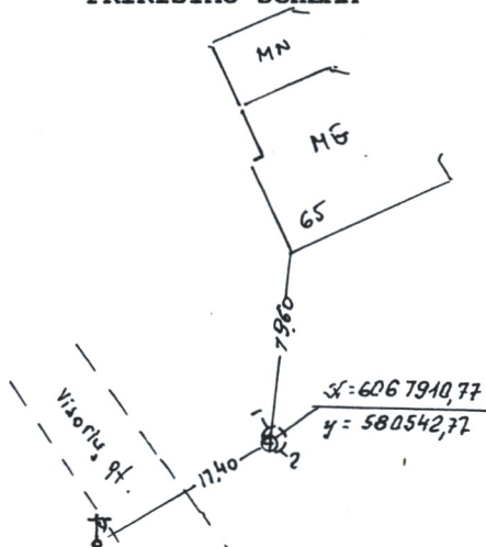
PRIRIŠIMO SCHEMA
