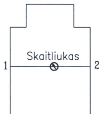
ŠULINIO PJŪVIAI (Matmenys duoti m)
